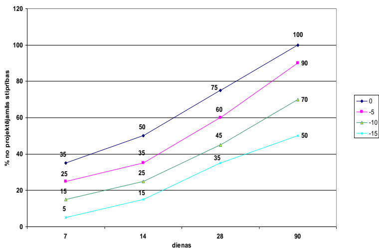
Stiprības diagramma cietējot zemās temperatūrās betonam ar pretsala piedevu AF.
