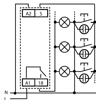
conexiune prin 4 conductori
