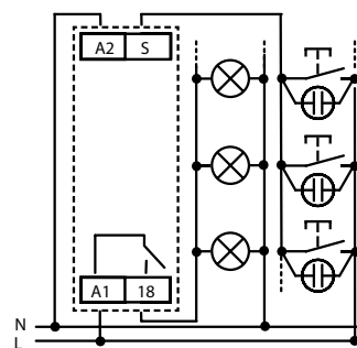
conexiune prin 4 conductori
