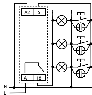
4-vodičové pripojenie
